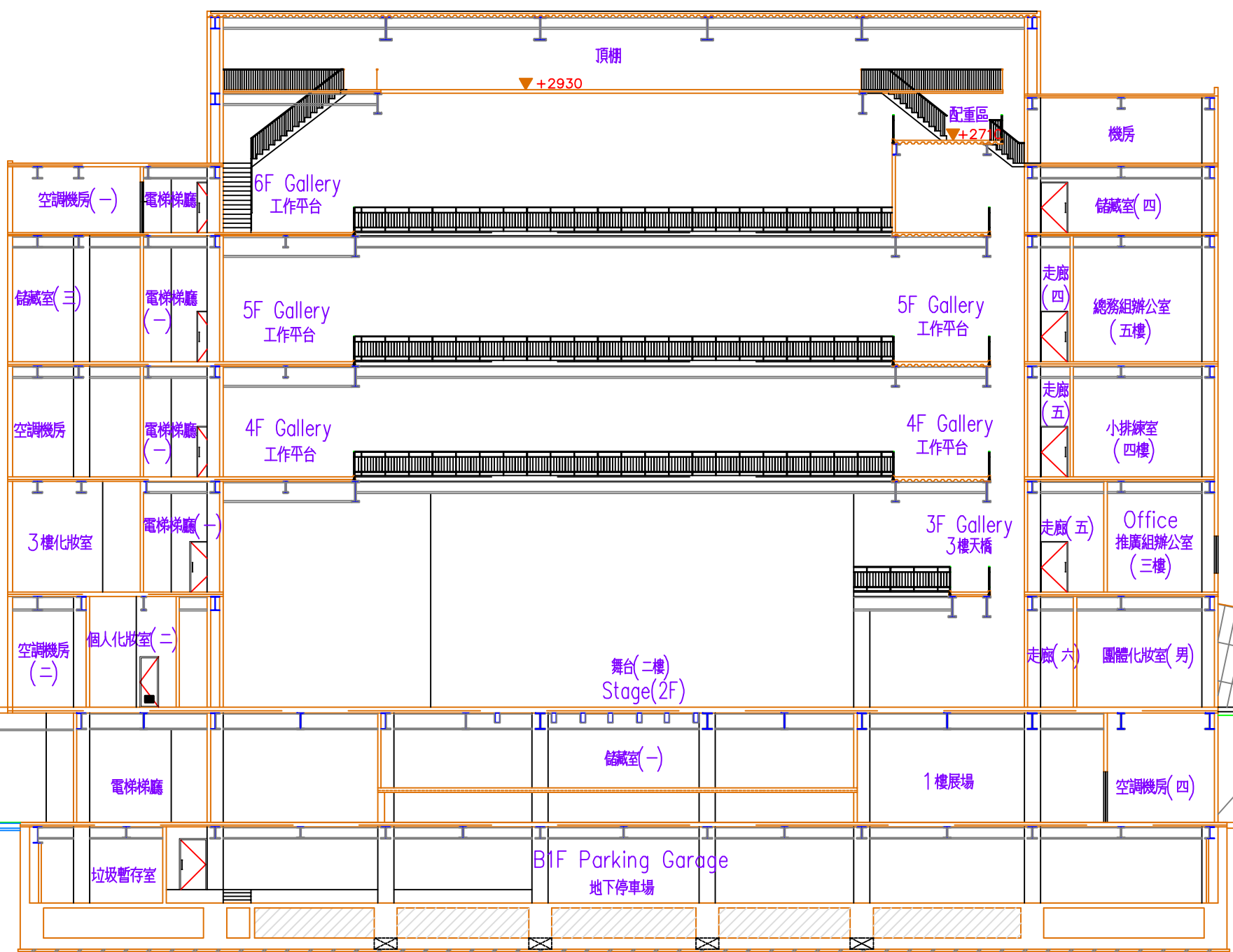
3 橫向總剖面圖(三) Cross Section(3)
