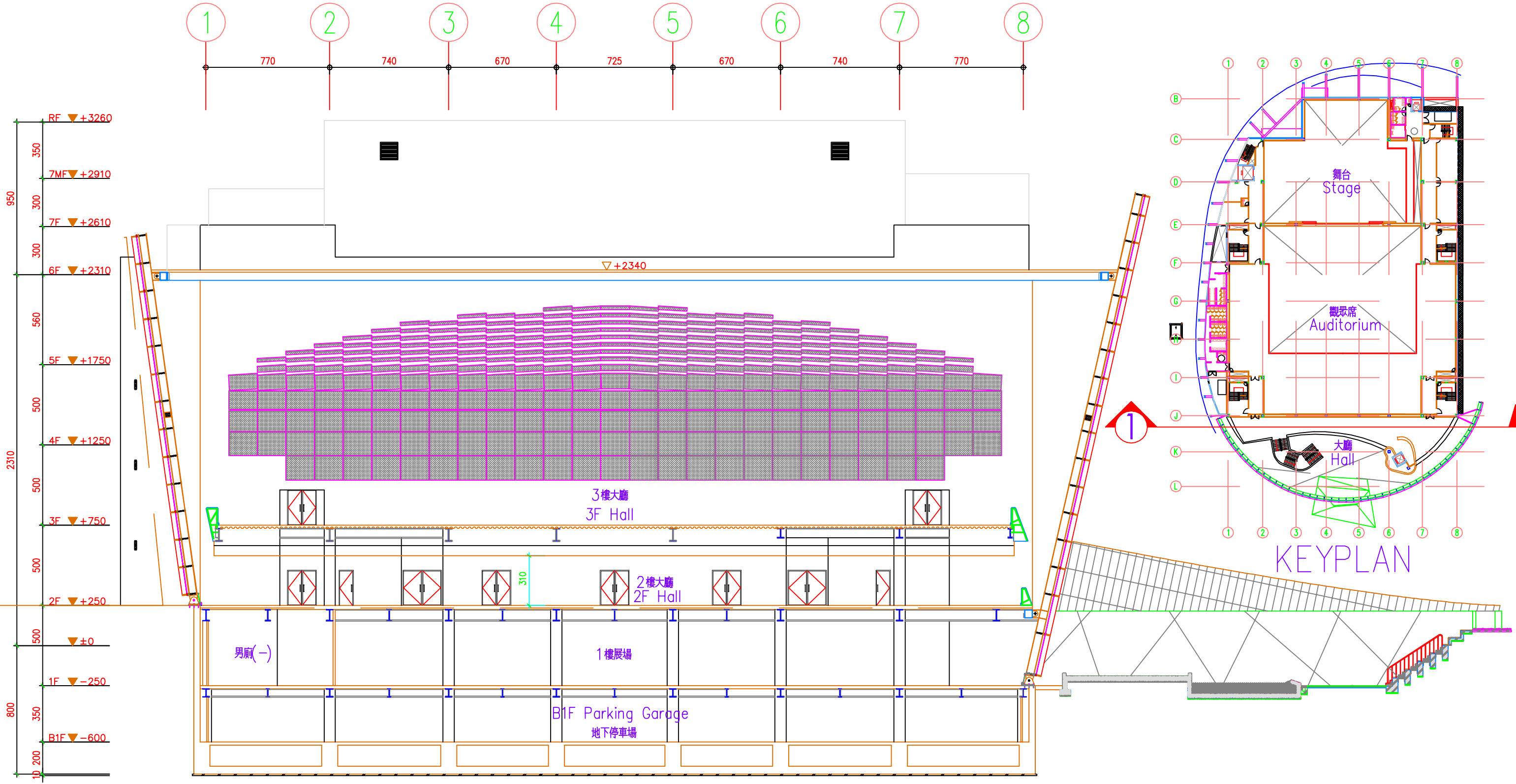
1 橫向總剖面圖(一) Cross Section(1)
