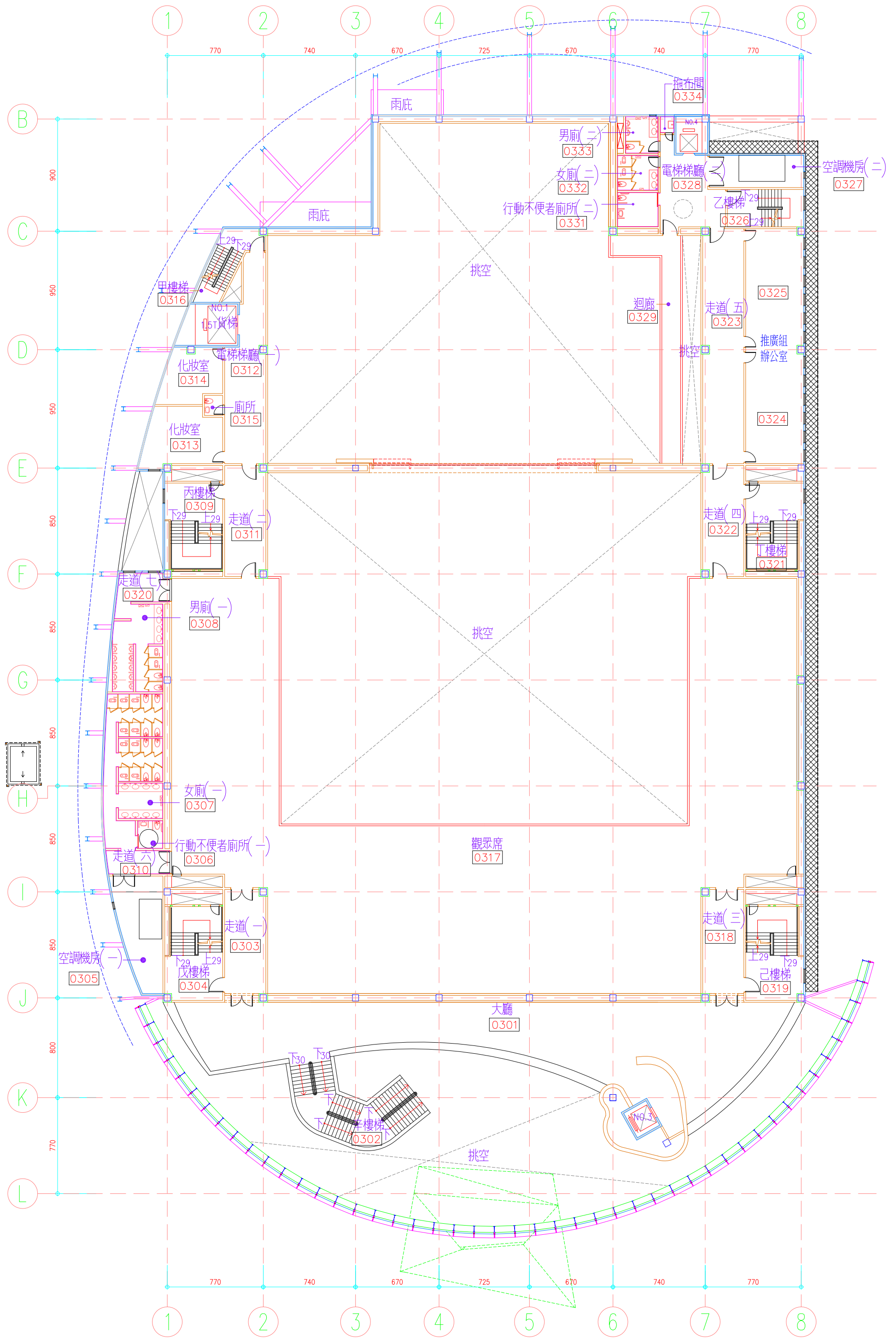
三層平面配置圖
